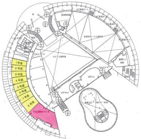
夢みなとタワー 2階平面図
